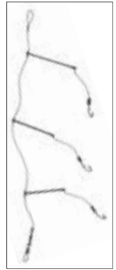
Albatros Patemonster met 3 afhouders Hoofdlijn: 0,50 mm Zijlijn: 0,45 mm Lengte: 90 cm
