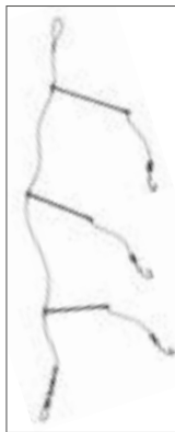
Albatros Klauwpatemonster met 3 afhouders Hoofdlijn: 0,50 mm Zijlijn: 0,45 mm Lengte: 90 cm
